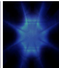
Multicusp plasma
